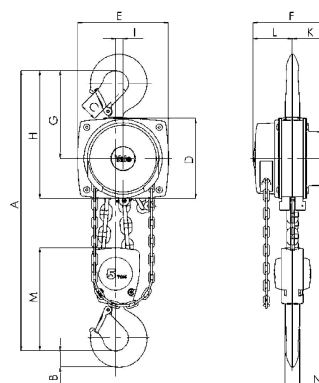
Modèle Yalelift 360, 5000 kg, 2 brins
