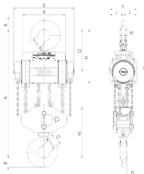
Modèle Yalelift 360, 20000 kg, 6 brins
