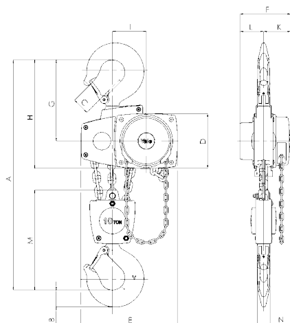
Modèle Yalelift 360, 10000 kg, 3 brins
