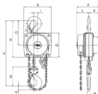
Modèle Yalelift 360, 500 - 3000 kg, 1 brin
